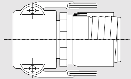
ACOPLE hembra
