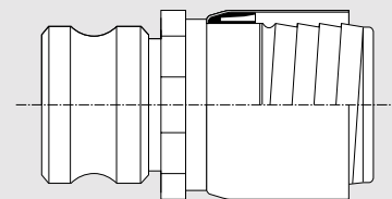
ADAPTADOR macho
